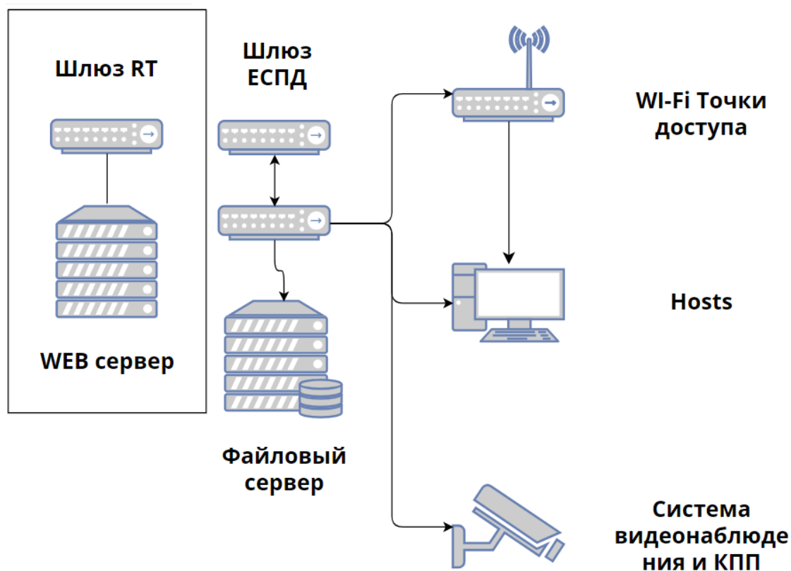
Схема локальной сети школы.
