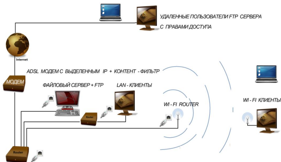
Схема локальной сети школы.
